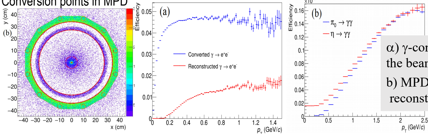
\eta \rightarrow \gamma\gamma \rightarrow (e^+e^-)(e^+e^-)
