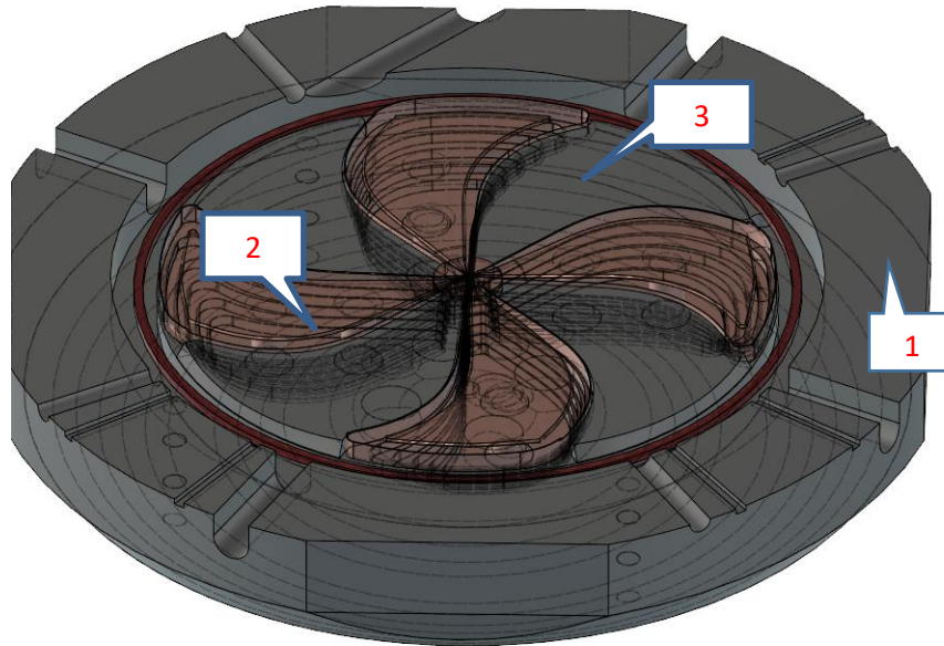
Рисунок 2. Магнитная и ускоряющая системы циклотрона SC230: 1 – ярмо, 2- дуанты и резонаторы, 3- сектора.
