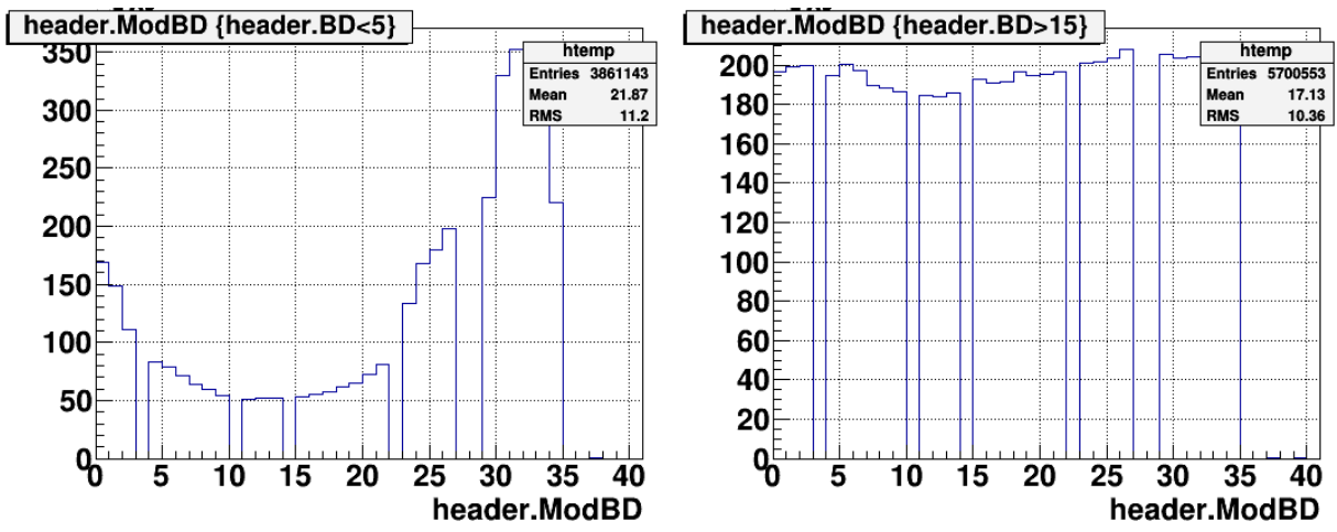
Рис. 2: Распределение по модулям в BD при разных множественностях. Cu@4GeV.
