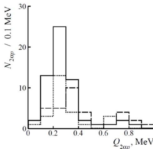
Рис. 3. Распределение числа 2\alpha\text{p} -троек N_{2\alpha\text{p}} по инвариантной массе Q_{2\alpha\text{p}} (< 1 \text{ МэВ}) в событиях когерентной диссоциации {}^{10}\text{C} \rightarrow 2\text{He}2\text{H} (сплошная) и диссоциации {}^{11}\text{C} \rightarrow 2\text{He}2\text{H} (точки) и {}^{10}\text{B} \rightarrow 2\text{HeH} (пунктир).
