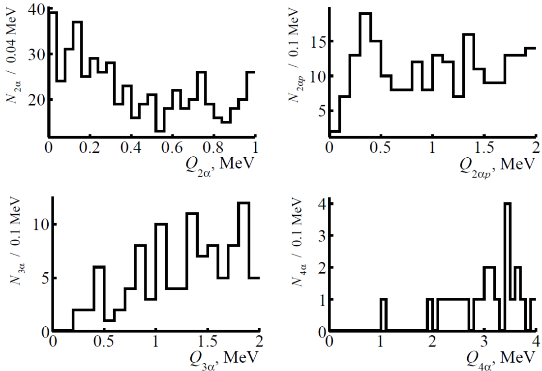
Рис. 8. Распределения всех комбинаций 2\alpha , 2\alpha p , 3\alpha и 4\alpha из событий фрагментации ядер {}^{197}\text{Au} при 10.7 \text{ A ГэВ} по инвариантным массам Q_{2\alpha} (a), Q_{2\alpha p} (b), Q_{3\alpha} (c) и Q_{4\alpha} (d) в областях из малых значений.
