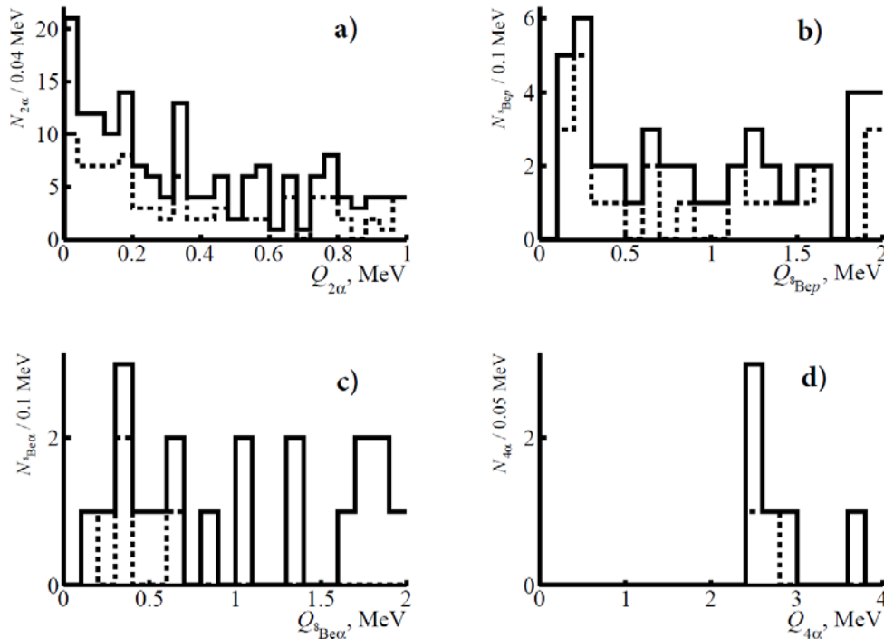
Рис. 7. Распределения всех комбинаций 2\alpha , 2\alpha p , 3\alpha и 4\alpha из событий фрагментации ядер ^{28}\text{Si} при 14.6 А ГэВ по инвариантным массам Q_{2\alpha} (a), Q_{2\alpha p} (b), Q_{3\alpha} (c) и Q_{4\alpha} (d) в областях их малых значений по данным без выборки (точки) и недавним измерениям при ускоренном поиске (добавлено, сплошная линия).
