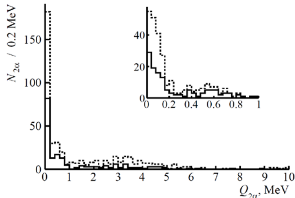
Рис. 2. Распределение числа 2\alpha -пар N_{2\alpha} по инвариантной массе Q_{2\alpha} в 500 событиях диссоциации {}^9\text{Be} \rightarrow 2\alpha (пунктир) при 1.2 \text{ A ГэВ} и в 198 “белых” звездах из их числа (сплошная); на вставке увеличенная часть Q_{2\alpha} < 1 \text{ МэВ} .
