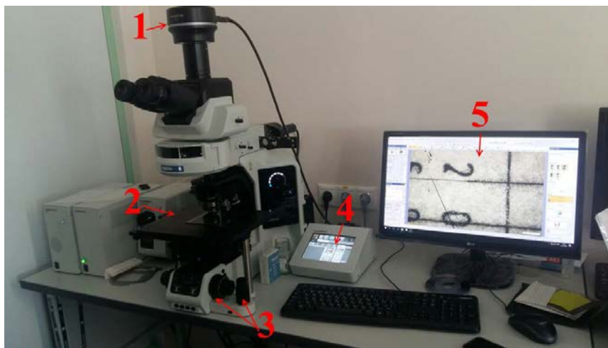
Рис. 11. Микроскоп ВХ63. Отмечены: 1) цифровая камера DP74, 2) моторизованный предметный столик, 3) джойстики управления фокусом и перемещением предметного столика в плоскости ХОУ, 4) блок управления микроскопом, 5) ПК для работы с получаемым изображением.
