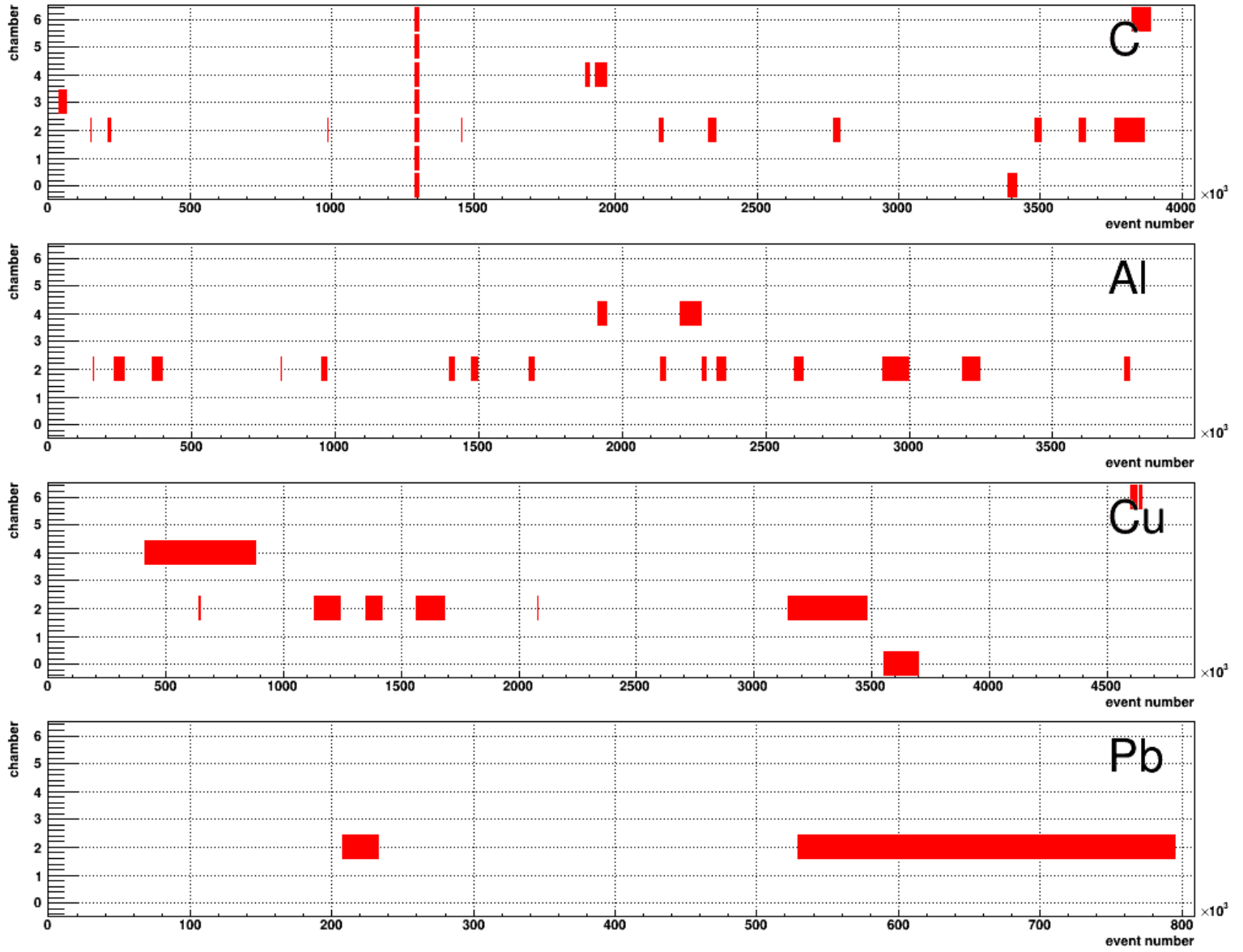
Рис. 1: T=4 GeV
