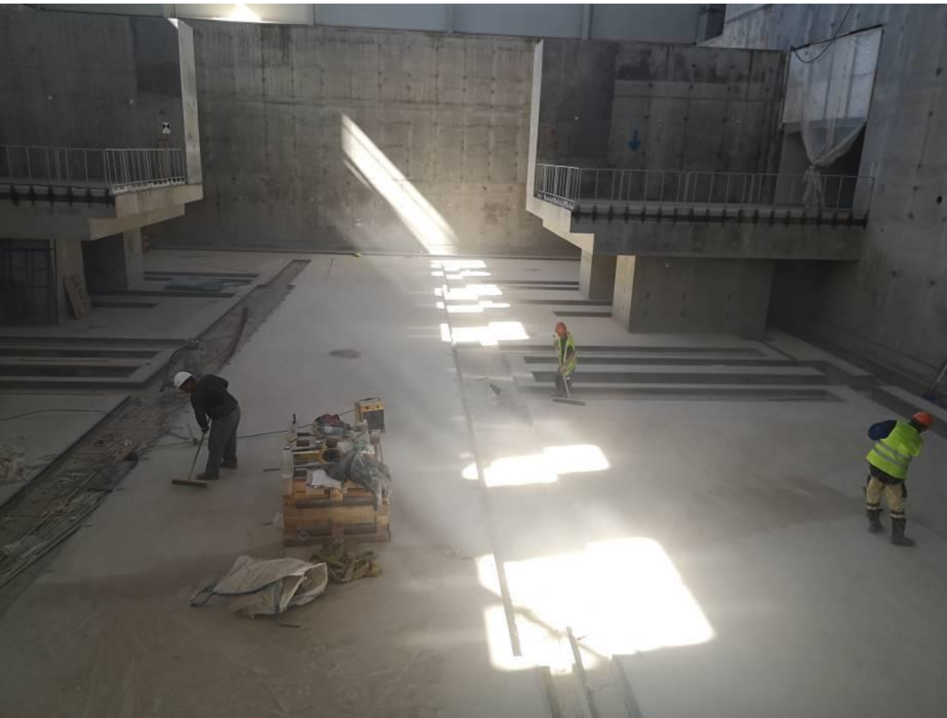
Шлифовка залитого бетона закончена. Идёт уборка, подготовка приямка зала к заливке эпоксидной смолой
