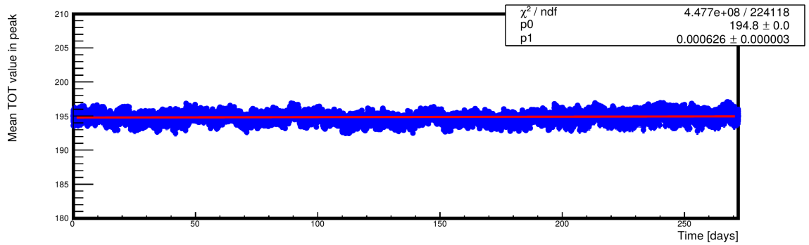
Рис. 12: Изменение положения фотопика источника ^{241}\text{Am} в зависимости от времени.
