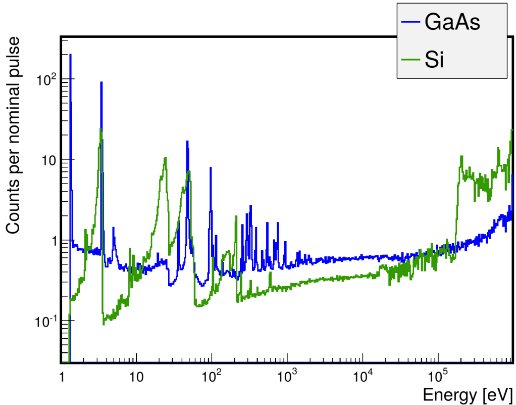
Рис. 18: Спектр нейтронов в детекторах Timex с сенсорами из кремния и арсенида галлия.
