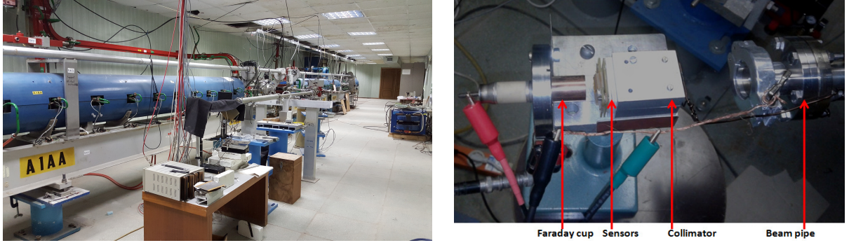
Рис. 2: Канал вывода пучка ускорителя Линак-200 и установка для облучения пэд-овых детекторов.
