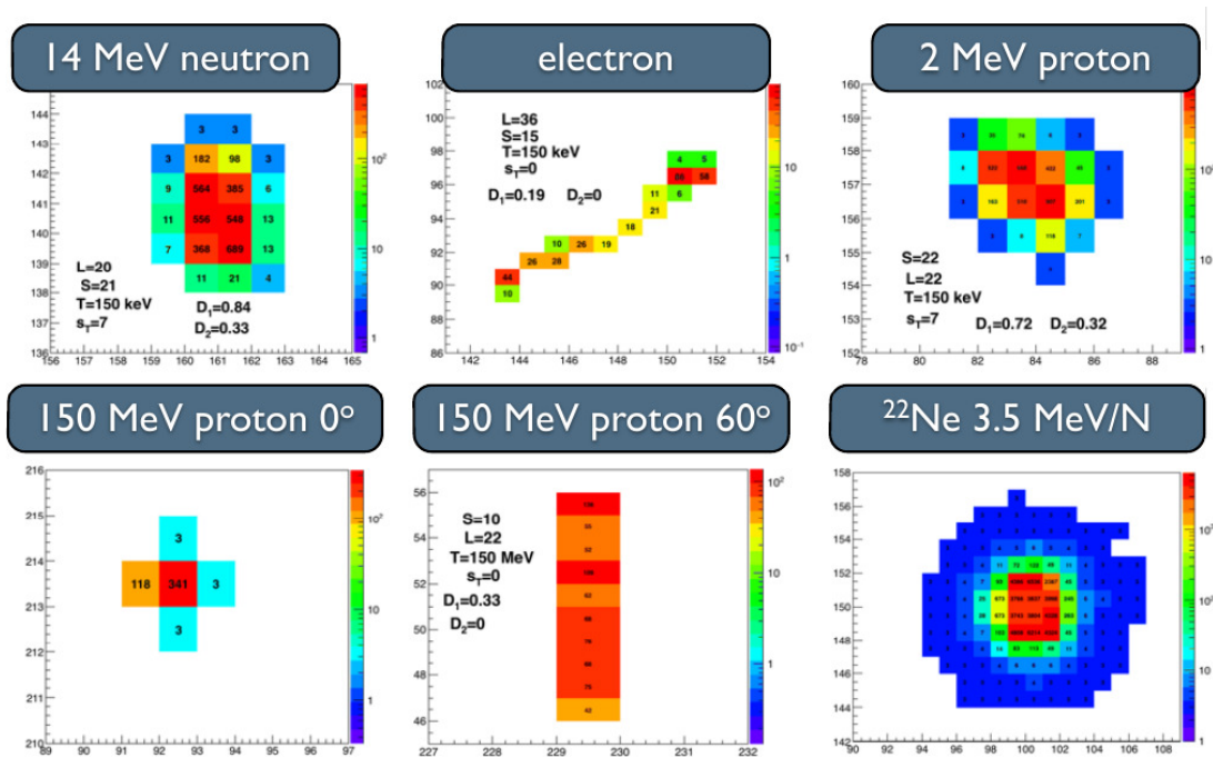
Рис. 16: Типичные кластеры, образуемые в детекторах Timex различными типами частиц.
