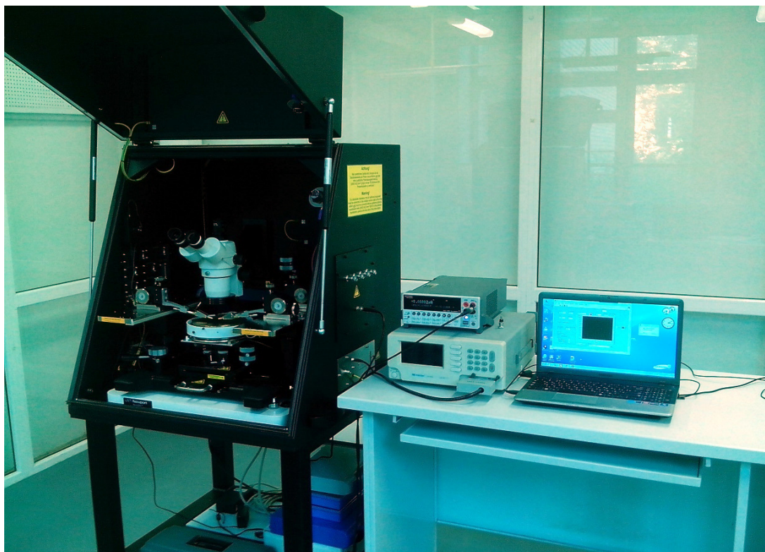
Рис. 21: Испытательный стенд на основе зондовой станции Cascade Microtech EPS150TESLA для изучения свойств полупроводниковых материалов.
