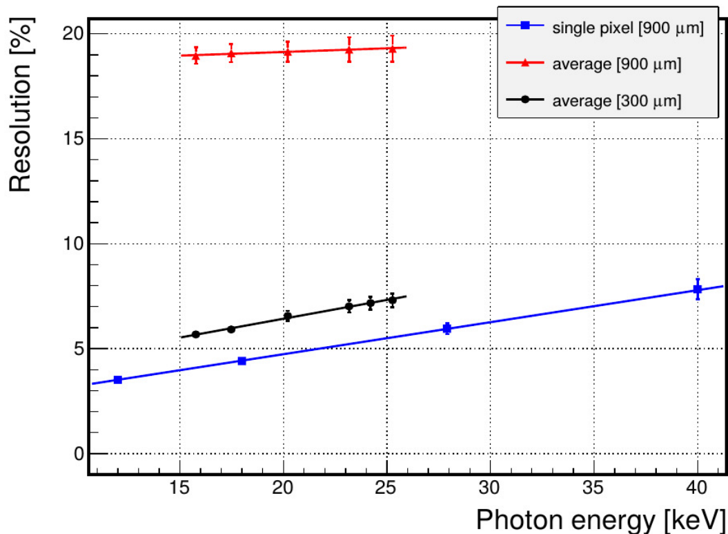
Рис. 15: Зависимость энергетического разрешения детектора (выраженная в процентах от измеренной энергии) от энергии фотона.
