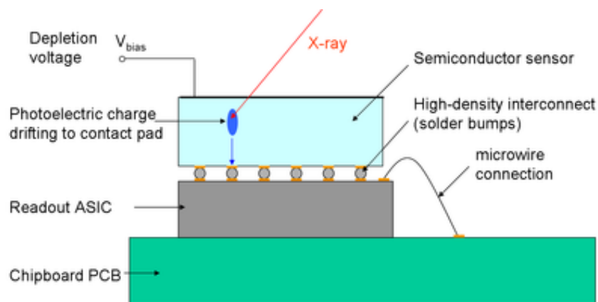
Рис. 1: Типичная схема гибридного пиксельного детектора.
