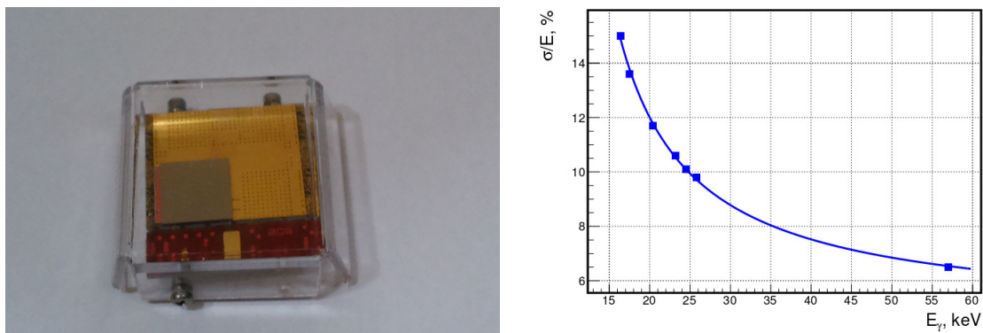
Рис. 10: Общий вид и энергетическое разрешение пиксельного детектора Timerix с арсенидогаллиевым сенсором толщиной 1 мм.
