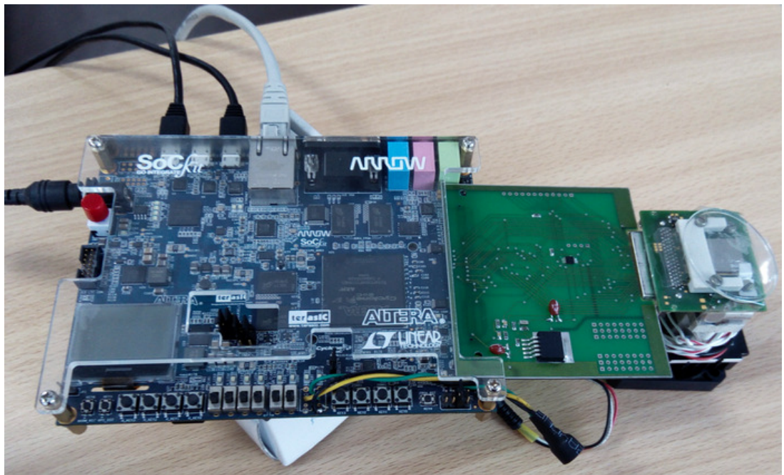
Рис. 26: Прототип электроники считывания для детектора семейства Medipix.
