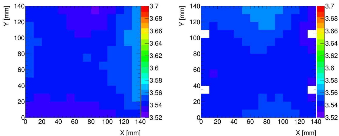
Рис. 8: Результаты измерения формы поверхности пластин вольфрамового поглотителя FCAL. Показано расстояние до поверхности пластины в мм относительно плоскости основания для двух сторон поглотителя.
