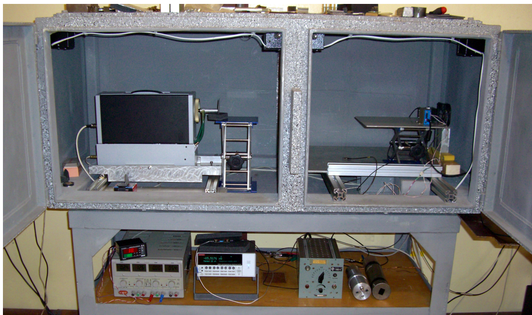
Рис. 20: Измерительный стенд “Калан”.
