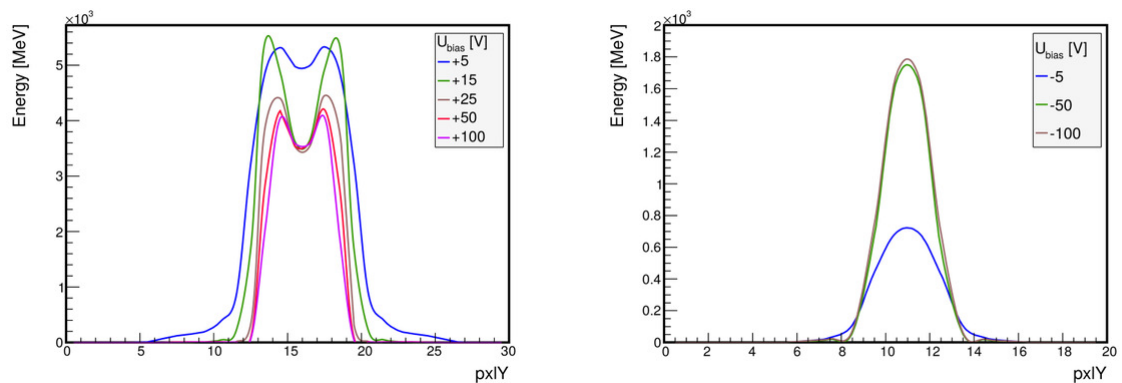
Рис. 19: “Вулкан-эффект” в кремниевом (слева) и арсенидогаллиевом (справа) детекторе Timerix при облучении ионами неона с энергией 158 МэВ.
