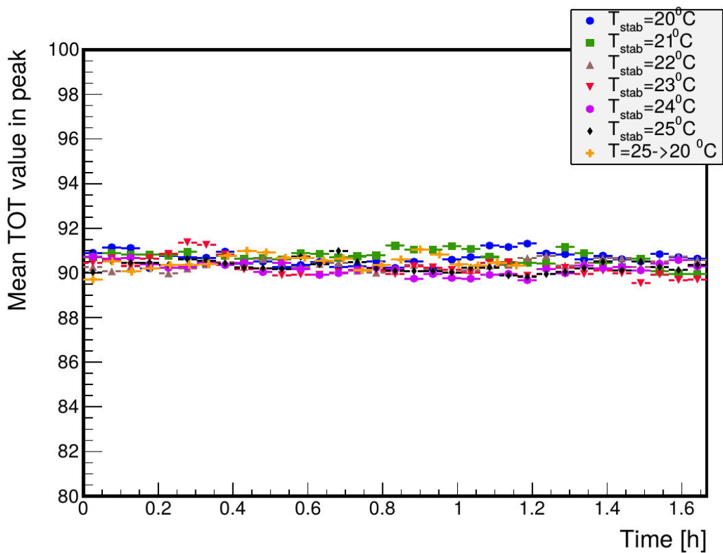
Рис. 13: Стабильность положения фотопика источника ^{241}\text{Am} при различной температуре.
