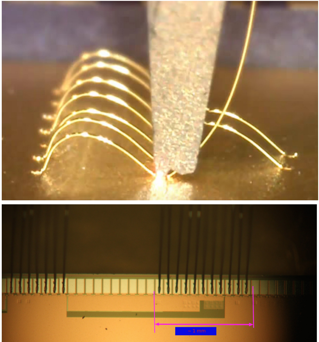
Рис. 24: Пример создания микропроволочных соединений методом “клин-клин” (вверху) и пример соединений микросхемы Medipix с платой считывания.
