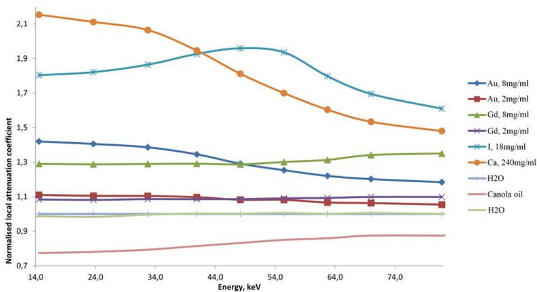
Рис. 28: Зависимость ЛКО от энергии для различных веществ (ЛКО отнормирован на ЛКО воды)
