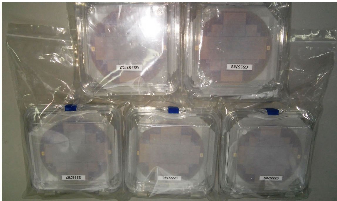
Рис. 9: Опытные образцы сенсорных пластин диаметром 102 мм, изготовленные в рамках проекта GALAPAD-2.
