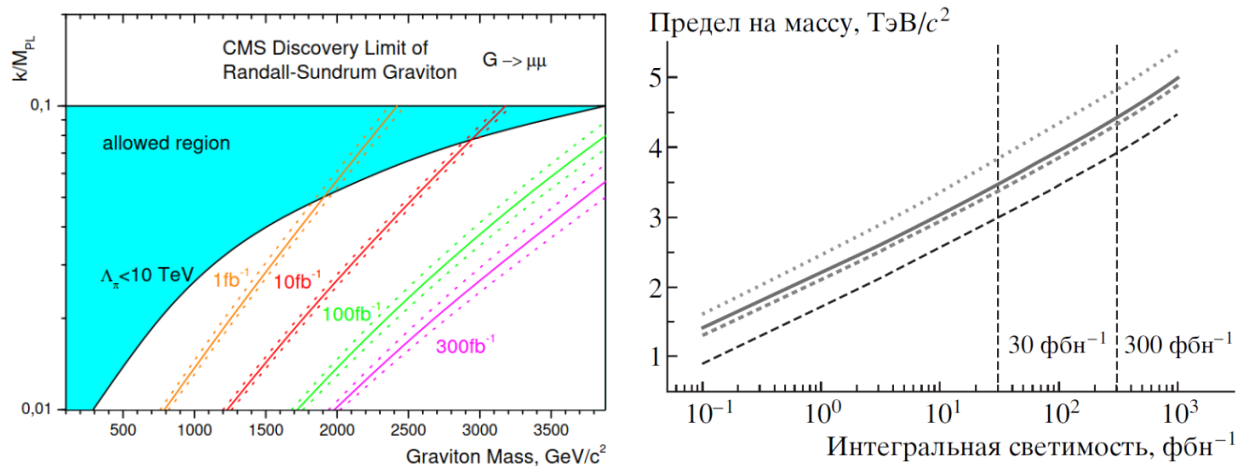
Рис. 3. Левый – ожидаемые экспериментальные ограничения в пространстве модельных параметров [3]. Правый – верхний предел, соответствующий статистической значимости более 5\sigma для разных значений интегральной светимости, на массу Z' бозона при распаде на \mu^+\mu^- для (кривые сверху вниз) SSM, \chi -модели, ALRM и \psi -модели для pp -соударений при \sqrt{s} = 14 ТэВ [4].
