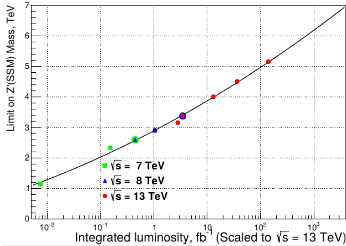
Рис. 10. Наблюдаемые при энергии в с.д.м. 7, 8 и 13 ТэВ массовые пределы для гипотетического калибровочного бозона Z' в модели SSM в зависимости от интегральной светимости [23].
