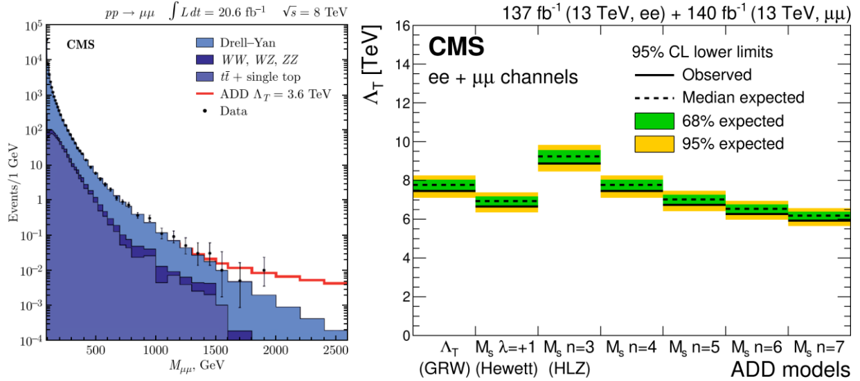
Рис. 11. Левый – распределение числа событий по инвариантной массе димюонов в конечном состоянии, полная статистика первого сеанса работы LHC \sqrt{s} = 8 ТэВ [17]. Правый – верхний предел (95% C.L.) на масштаб многомерной гравитации в рамках различных схем перенормировки GRW ( \Lambda_T ) и HLZ ( M_S ) при \sqrt{s} = 13 ТэВ [34]. Результаты для схемы HLZ приведены в зависимости от числа дополнительных измерений n .
