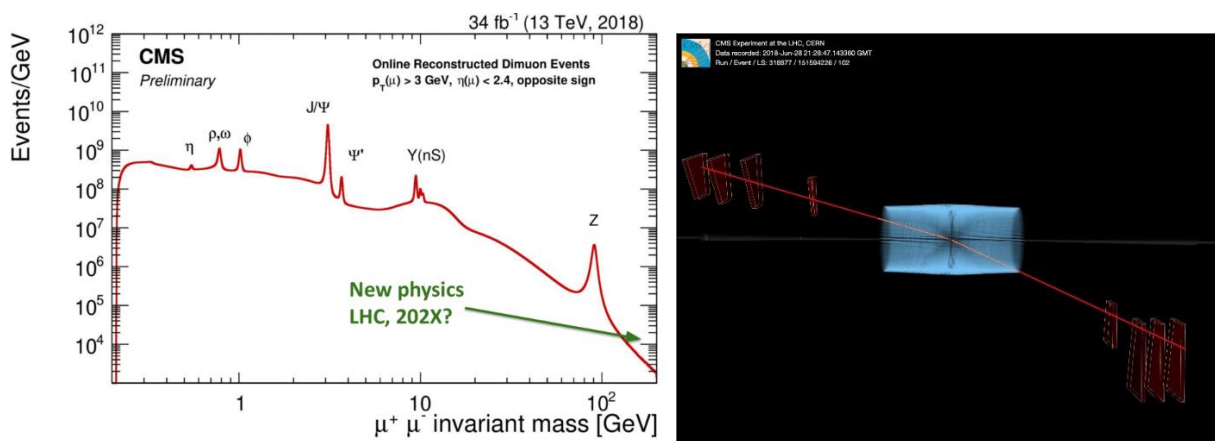
Рис.1. Левый – Спектр инвариантных масс димюонов с характерными пиками в распределении, соответствующими открытым в ускорительных экспериментах частицам. Правый – визуализация события-кандидата с наивысшей массой из числа зарегистрированных CMS дилептонов со значением инвариантной массы 3.34 ТэВ/c 2 .
