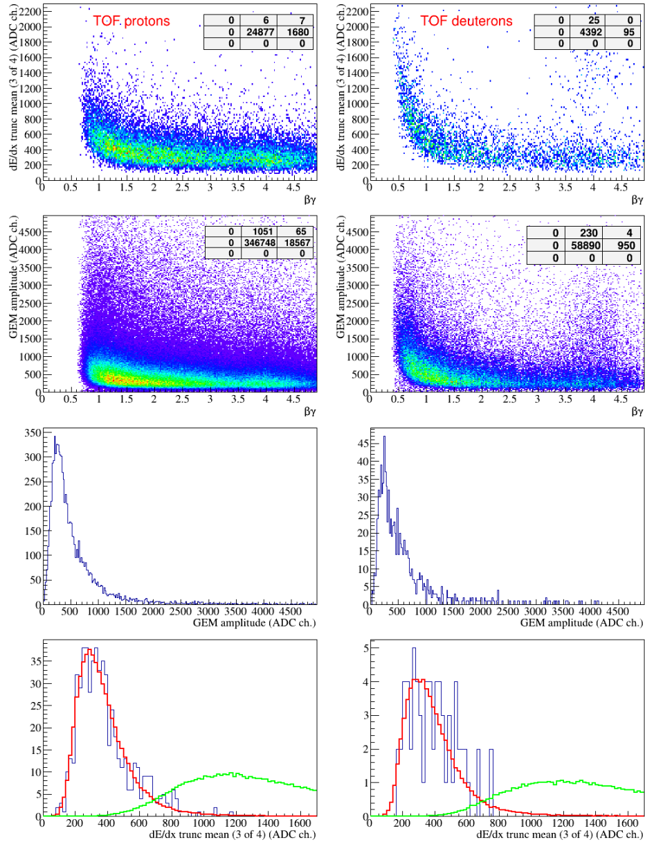
Рис. 17: Оценка энергетических потерь 4-хитовых треков и потери в плоскости GEM для треков, отобранных в TOF-700, как протоны и дейтроны. Нижний ряд: потери трека и разыгрыш из потерь в плоскостях для 2.5 < \beta\gamma < 2.6 .
