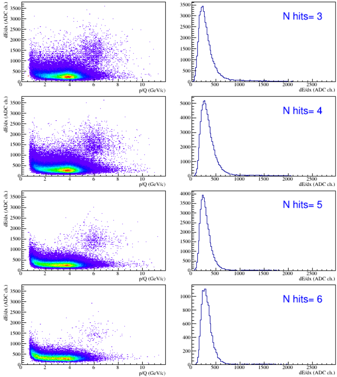
Рис. 14: Protons: 0.5 < m^2 < 1.2 ( \text{GeV}/c^2 ) 2 . Справа: 4 < p/Q < 9 GeV/c.
