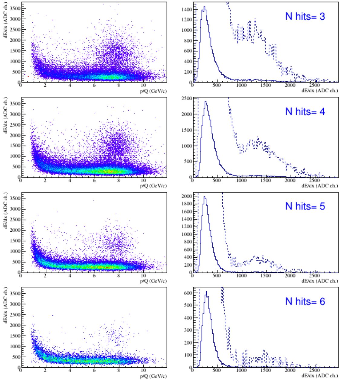
Рис. 16: d and {}^4\text{He} : 2.5 < m^2 < 4.5 ( \text{GeV}/c^2 ) ^2 . Справа: 4 < p/Q < 9 \text{GeV}/c . Пунктир - гистограмма умножена на 20.
