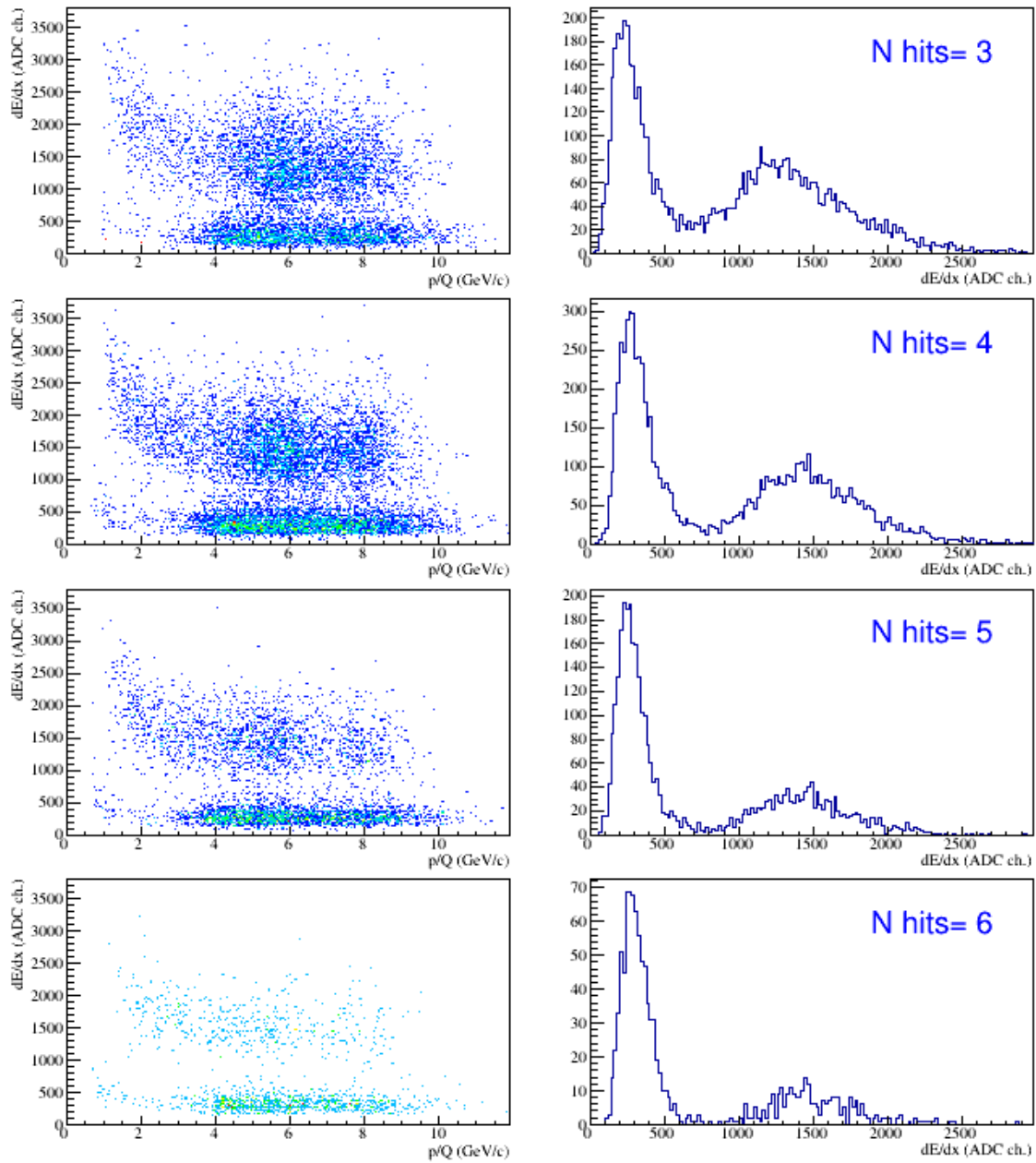
Рис. 15: {}^3\text{He} : 1.5 < m^2 < 2.3 ( \text{GeV}/c^2 ) 2 . Справа: 4 < p/Q < 9 \text{GeV}/c . Похоже, {}^4\text{He} погибает в этот коридор.
