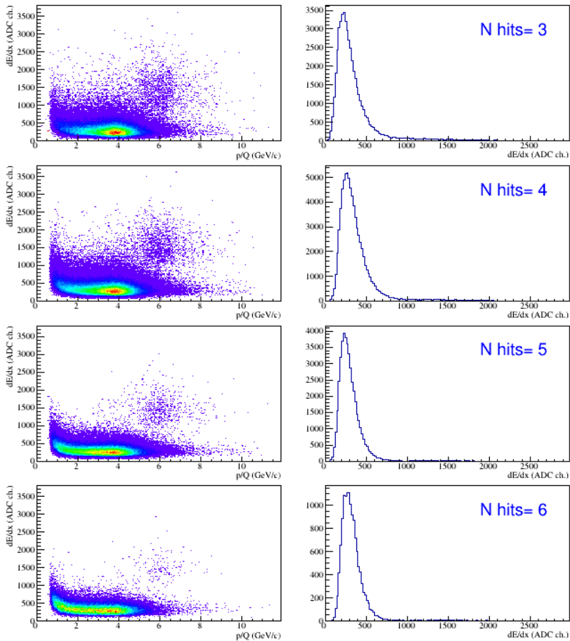
Рис. 15: Protons: 0.5 < m^2 < 1.2 ( \text{GeV}/c^2 ) 2 . Справа: 4 < p/Q < 9 GeV/c.
