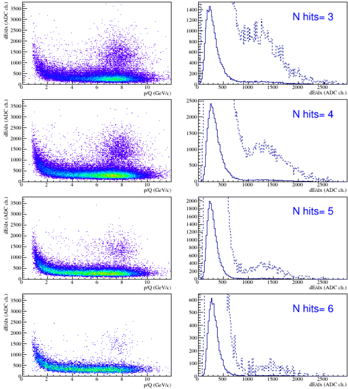
Рис. 17: d and {}^4\text{He} : 2.5 < m^2 < 4.5 \text{ (GeV}/c^2)^2 . Справа: 4 < p/Q < 9 \text{ GeV}/c . Пунктир - гистограмма умножена на 20.
