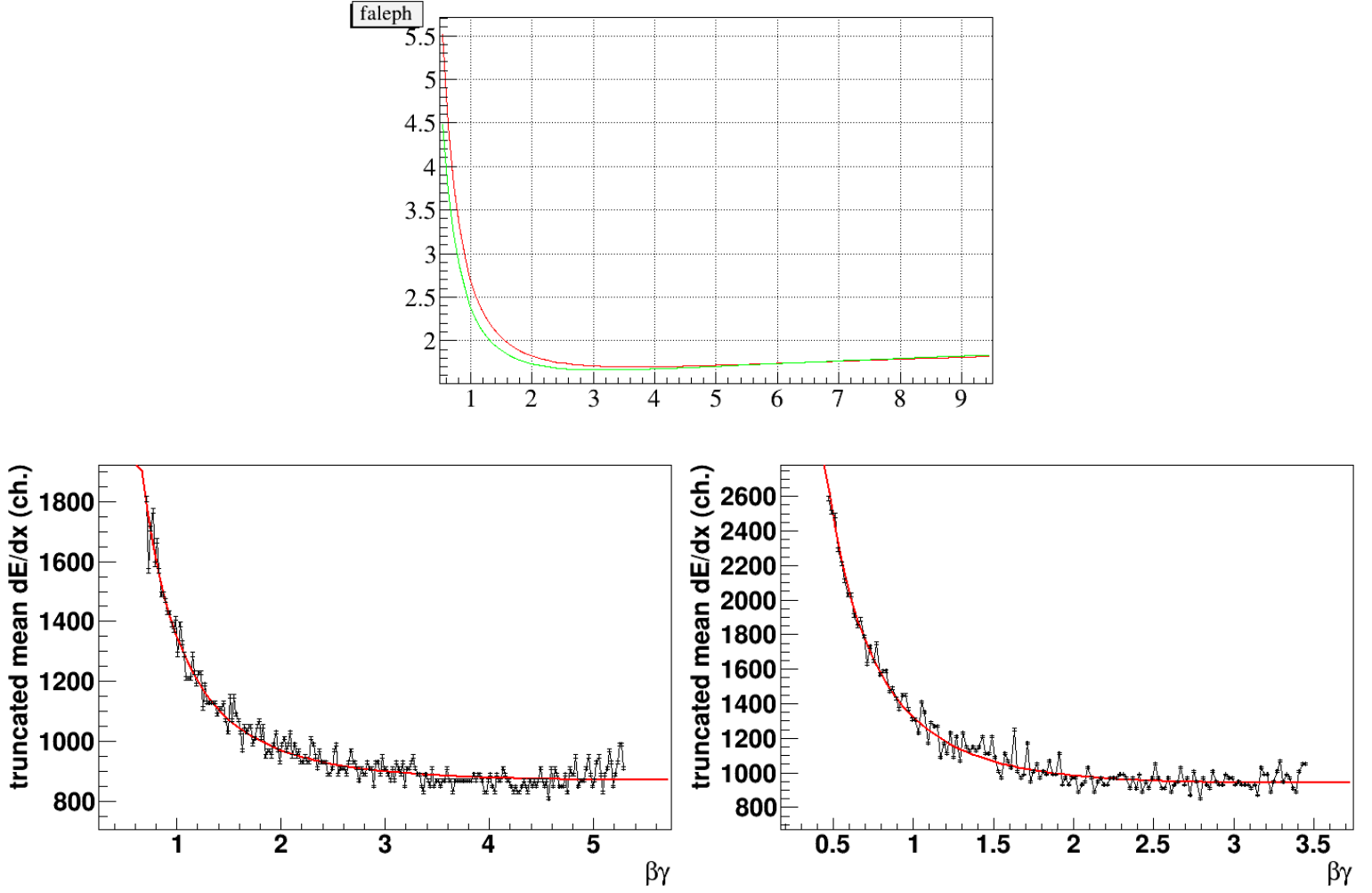
Рис. 28: Q1TM.C для 1% p и d . p_{beam}/m_p=4.2957 . Фит ALEPH.
