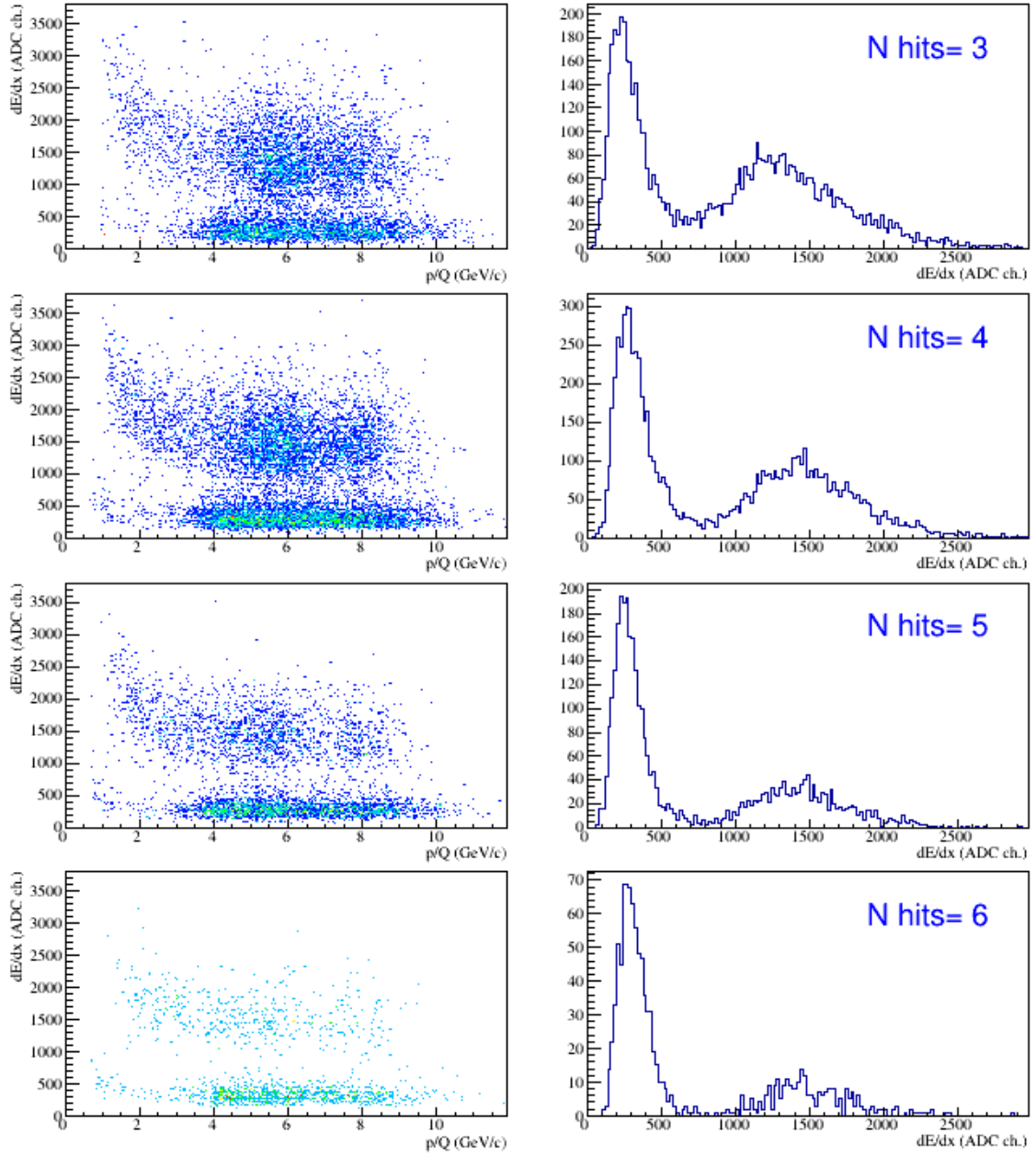
Рис. 16: ^3\text{He} : 1.5 < m^2 < 2.3 \text{ (GeV/c}^2\text{)}^2 . Справа: 4 < p/Q < 9 \text{ GeV/c} . Похоже, ^4\text{He} погибает в этот коридор.
