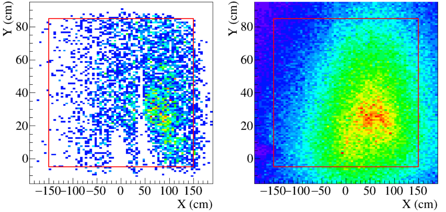
Рис. 10: Попадание в TOF700 z \equiv 700 , |x| < 150 , -5 < y < 85 .
