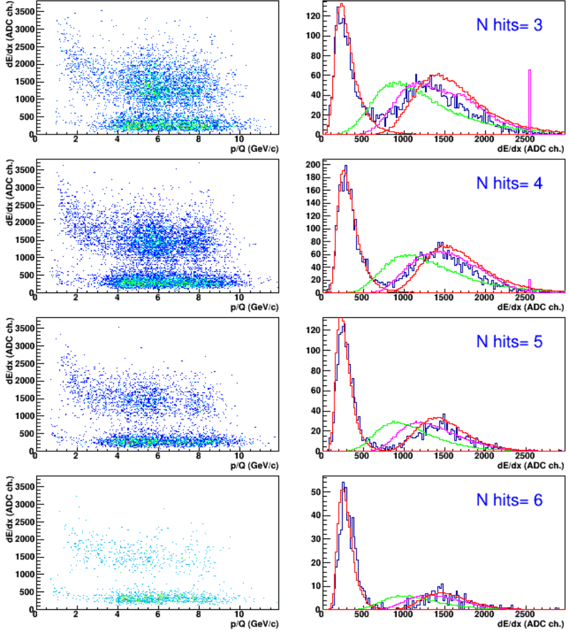
Рис. 19: {}^3\text{He} : 1.5 < m^2 < 2.3 \text{ (GeV/c}^2\text{)}^2 . Справа: 4 < p/Q < 7 \text{ GeV/c} . Зеленый - A_d = 4 A_p , сиреневый - A_d = \text{Min}(4 \cdot (A_p + 70), 2548) , красный - A_d = \sum_4 A_p .
