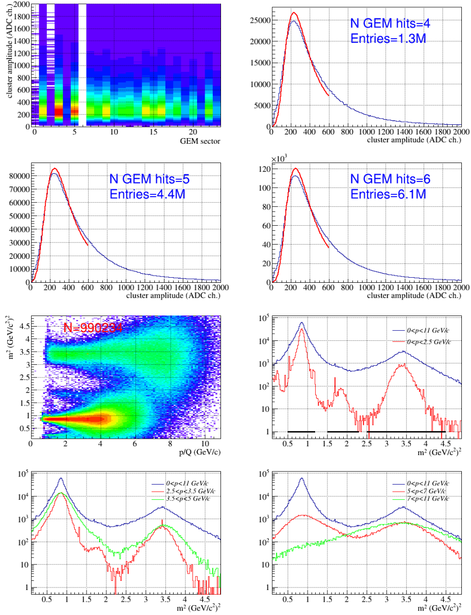
Рис. 13: Верх: Амплитуды GEM после коррекций ( N_{PVT_r} \leq 2 , |Z_{PV}| < 5 см, b_{imp} < 0.3 см, goodGemArea). Ниж: m^2 vs p . m^2 пределы идентификации: \pi : 0.1-0.35); tofPid=1; p : 0.5-1.2; ^3\text{He} : 1.5-2.3; \text{He} : 2.5-4.5.
