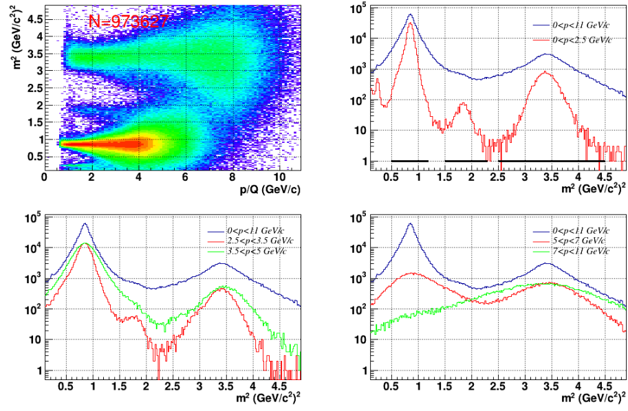
Рис. 14: m^2 vs p . m^2 пределы идентификации: \pi : 0.1-0.35); tofPid=1; p : 0.5-1.2; {}^3He : 1.5-2.3; He : 2.5-4.5. Выброшен run 4548 с повторяющимися массами.
