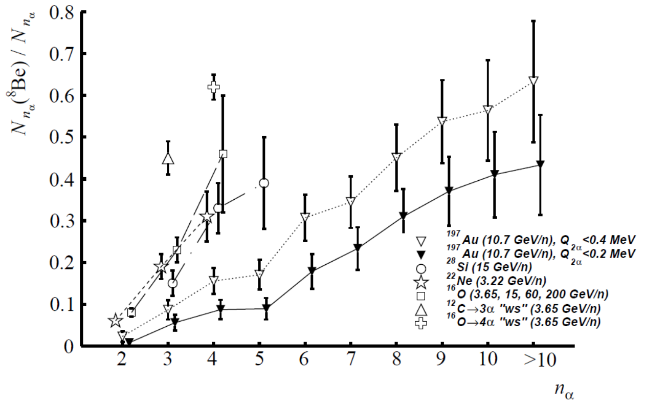
Рис. 6. Зависимость относительного вклада распадов N_{n_\alpha}({}^8\text{Be}) в статистику N_{n_\alpha} событий с множественностью \alpha -частиц n_\alpha в релятивистской фрагментации ядер C, O, Ne, Si и Au [13]; отмечены "белые" звезды {}^{12}\text{C} \rightarrow 3\alpha и {}^{16}\text{O} \rightarrow 4\alpha (WS); для удобства точки несколько смещены от значений n_\alpha и соединены пунктиром.
