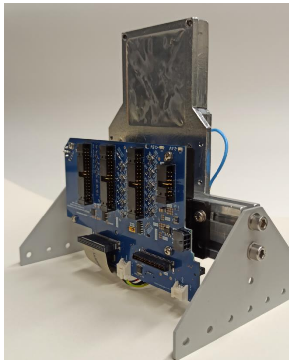
Рис.3 Координатная плоскость собрана на механической раме.
