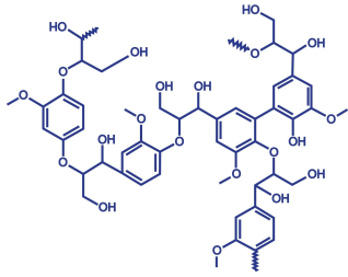
Lignin
