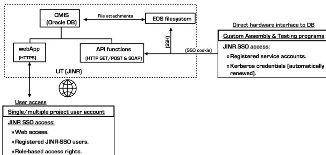
Рис. 1. Внедрение CMIS в LIT в ОИЯИ
