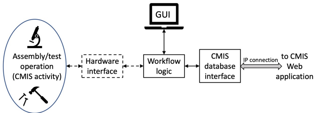
Рис. 5. Структура клиентского программного обеспечения CMIS.
