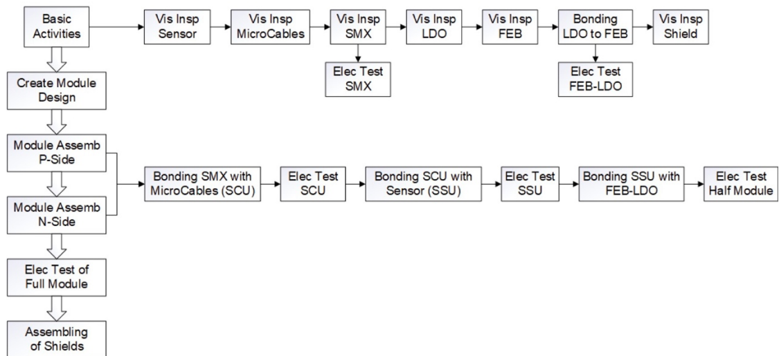
Рис. 4. Рабочий процесс сборки модуля детектора VM@N-STC.
