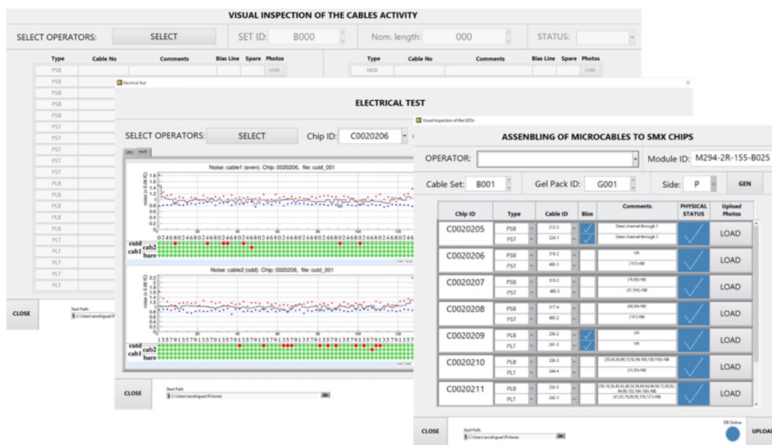
Рис. 6. Пример графического интерфейса на основе LabVIEW для регистрации операций сборки модулей VM@N-STС в CMIS
