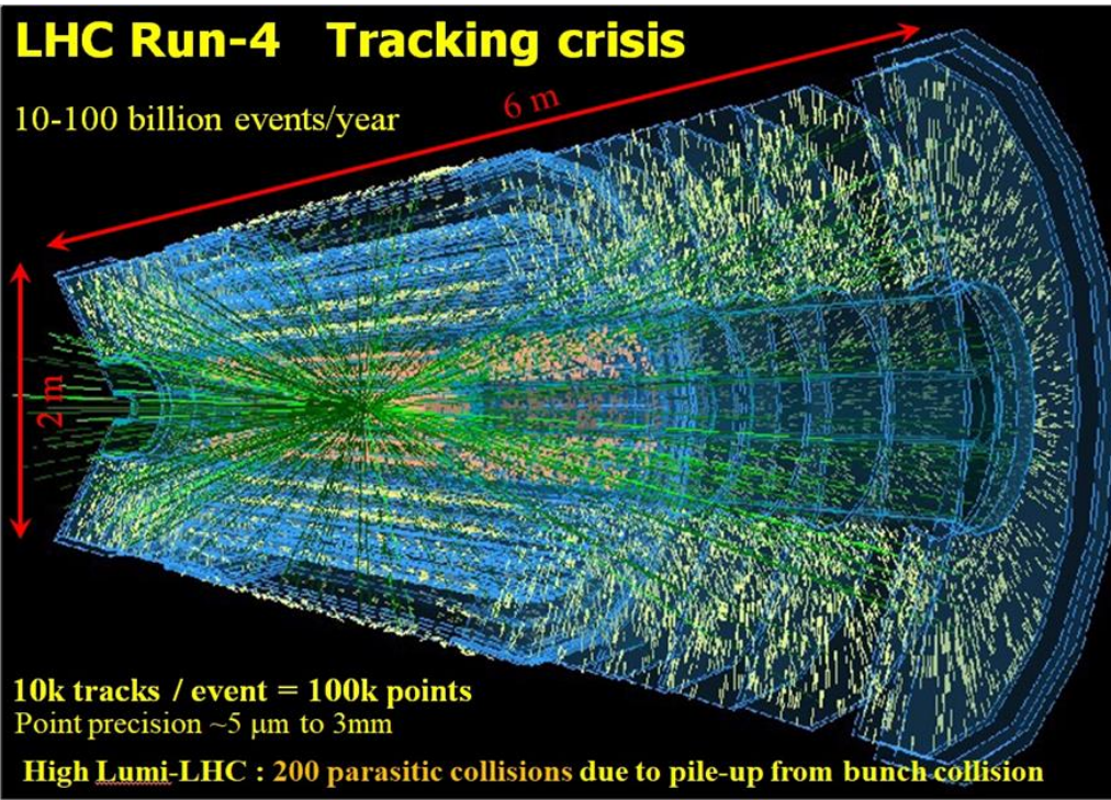
Модельное события в HL-LHC
