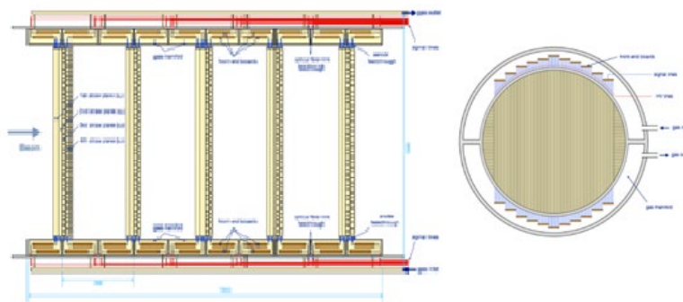
Рис. 5. Общая структура строу трекера (размеры строу увеличены в три раза для наглядности): (слева) вид сбоку; (справа) условный вид строу плоскости в поперечном сечении
