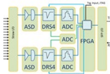
Рис. 14. Принципиальная схема платы ROESTI
