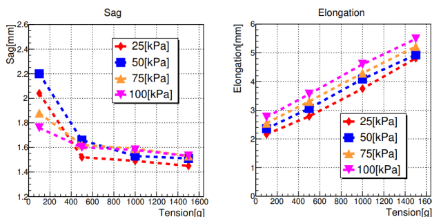
Рис. 10. Результаты исследования предварительного натяжения строу; (слева) провисание, определенное для различных перепадов давления в зависимости от приложенного натяжения, (справа) удлинения трубок
