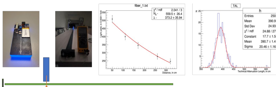
Рис. 51. Источник голубого света; источник света на расстоянии 320 см от фотоприемника; определение длины затухания для одного из волокон; распределение длин затухания
