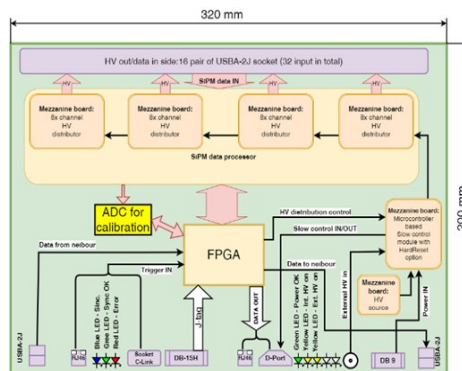
Рис. 50. Первый вариант FEBE, согласованный с коллегами из Новосибирска
