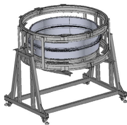
Рис. 29. Оснастка для сборки модуля с корпусом внутри
