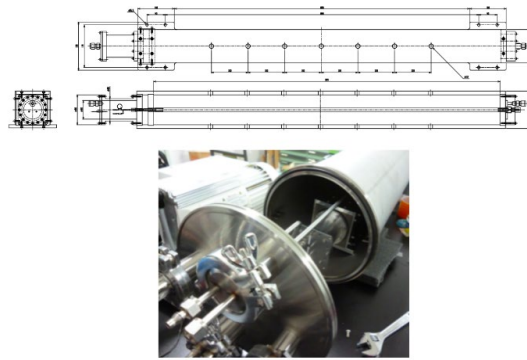
Рис. 16. Одноканальный прототип строу: (наверху) чертеж прототипа; (внизу) общий вид станда
