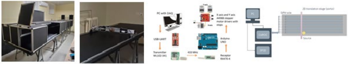
Рис. 52. «Черный ящик» с 2Д-порталом внутри; 2Д-портал на столе; блок-схема беспроводного управления 2Д-порталом для перемещения бета-источника; и блок-схема фронт-энд электроники для считывания данных
