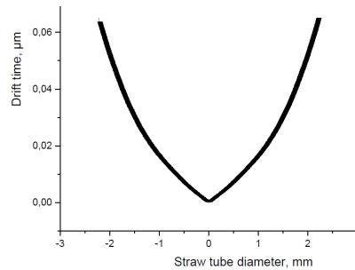
Рис. 56. Промоделированная R-T для строу-трубки диаметром 5 мм
