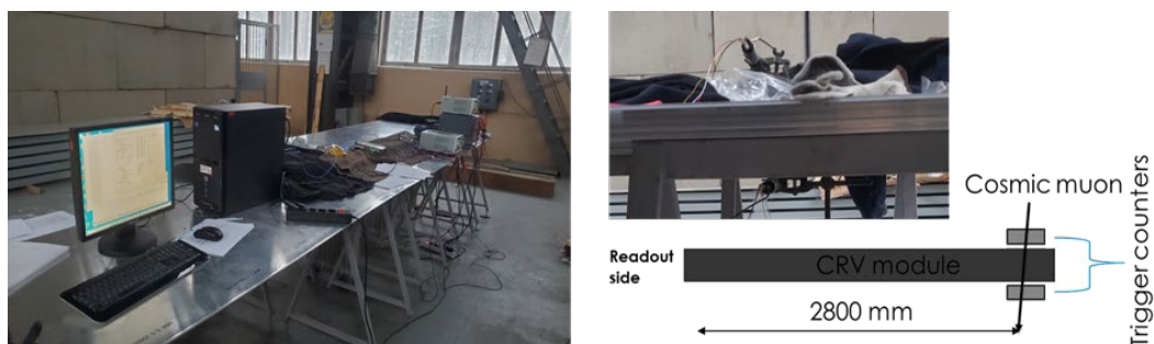
Рис. 55. Первые испытания модуля CRV с Метеором 32, проведенные в ОИЯИ
