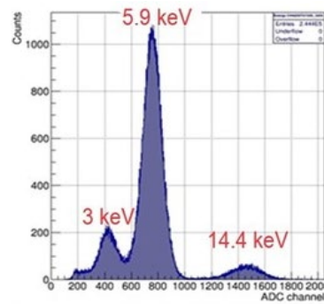
Рис. 23. Спектр, полученный на одноканальном прототипе (5 мм строу)
