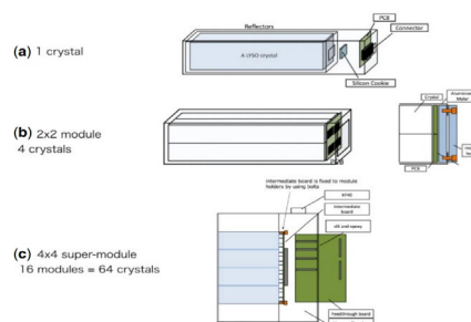
Рис. 39. Модульная структура ECAL: (а) 1 кристалл + 1 APD, (b) 2×2 кристаллический модуль; (c) супер модуль 4×4 (64 кристалла) и система считывания
