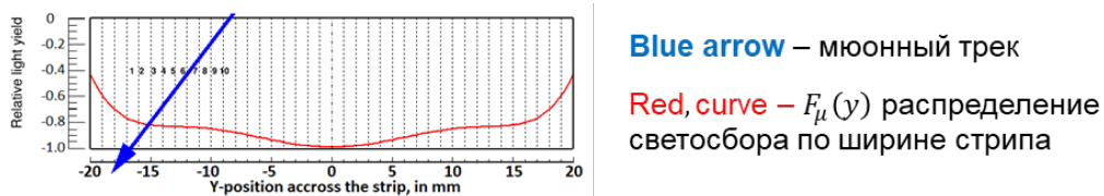
Рис. 46. Упрощенная модель подсчета светосбора
