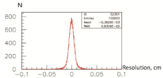
Рис. 58. Интегральное пространственное разрешение для строу-трубки
