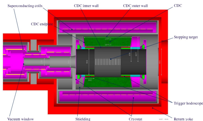
Рис. 3. Схематическое изображение CyDet
