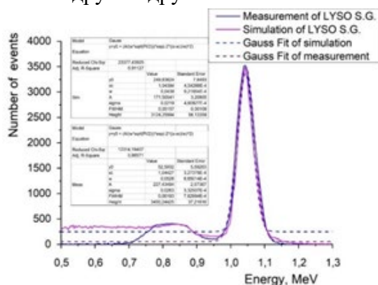
Рис. 60. Измеренный и промоделированный энергетические спектры LYSO:Ce кристалла, полученные для одинаковых условий (APD, 22Na: 1274 кэВ, отверстие коллиматора 0.5 мм)
