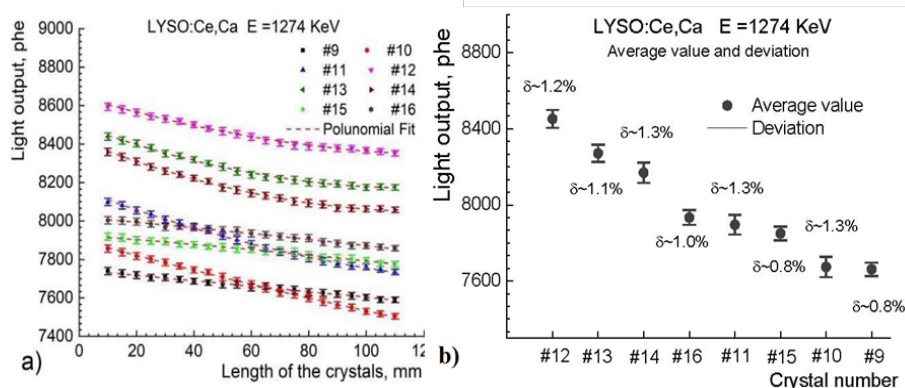
Рис. 33. а) Неоднородность световых выходов по длине LYSO:Ce,Ca кристаллов; б) Неоднородности откликов сцинтилляторов на энергии 1274 кэВ, нормированные на их среднее значение
