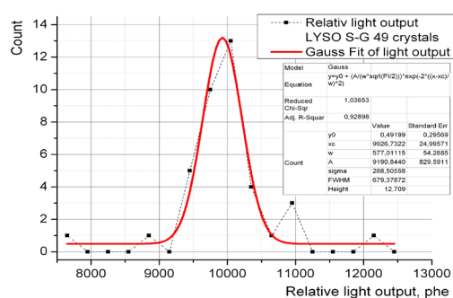
Рис. 31. Распределение относительного световыхода для 50 кристаллов LYSO:Ce
