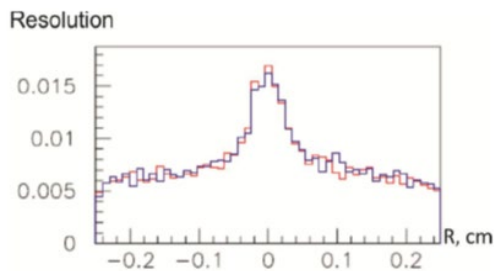
Рис. 57. Пространственное разрешение для строу по диаметру
