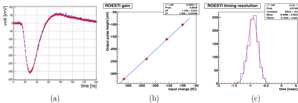
Рис. 15. Характеристики платы ROESTI: (а) выход тестового импульса, (б) калибровка усиления, (с) временное разрешение
