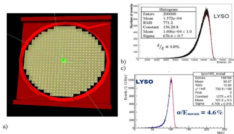
Рис. 61. Результаты моделирования калориметра: а) геометрия б) детектируемый энергетический спектр; в) результаты экспериментального измерения прототипа калориметра на электронном пучке ускорителя в Тохоку (Япония) в 2014 году
