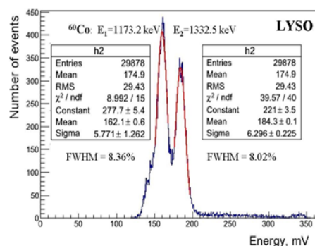
Рис. 35. Энергетический спектр, полученный с оптимальной оберткой: 2 слоя Тефлон и ESR пленка на источнике ^{60}\text{Co}
