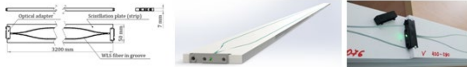
Рис. 43. Дизайн стрипа и фотография одного конца реального стрипа
