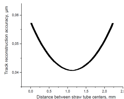
Рис. 59. Оценка точности восстановления трека
