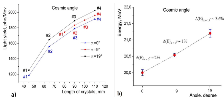
Рис. 37. Рис. Неоднородности отклика детектора для углов 0, 19 и 9^\circ , измеренная на космических мюонах а) распределения откликов сцинтилляторов прототипа по углу; б) средние значения и неоднородности отклика сцинтилляторов по углу
