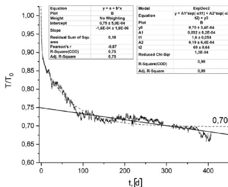
Рис. 12. Релаксация натяжения в длительном интервале времени
