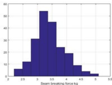
Рис. 8. Прочность шва строу 9.8 мм
