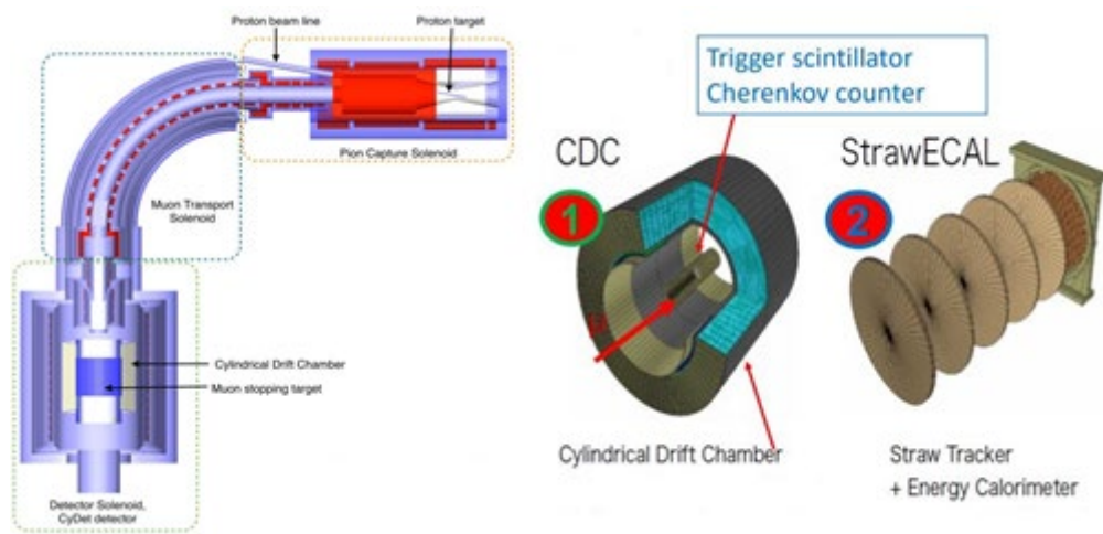
Рис. 2. Схематическое изображение Фазы-I COMET
