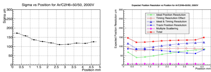
Рис. 21. Зависимость пространственного разрешения от положения трека: (слева) измеренная, (справа) промоделированная
