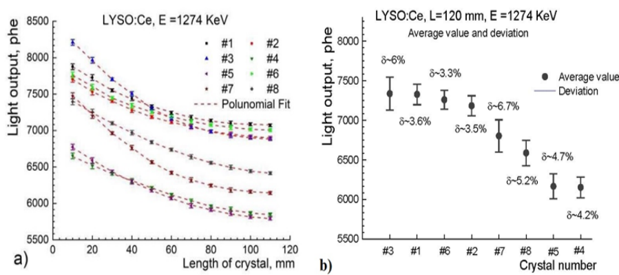
Рис. 32. а) Неоднородность световых выходов по длине LYSO:Ce кристаллов; б) Неоднородности откликов сцинтилляторов на энергии 1274 КэВ, нормированные на их среднее значение
