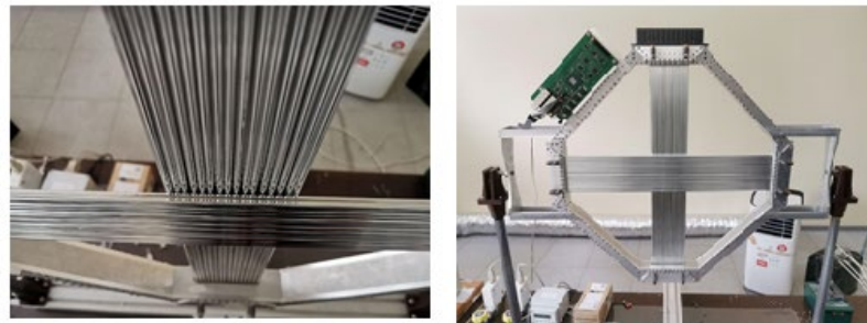
Рис. 24. Сборка 64-х канального мини прототипа модуля строу трекера
