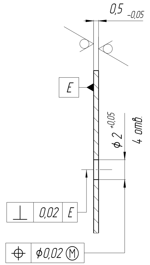
B-B (5:1)
