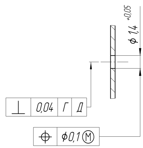
B-B (5:1)
