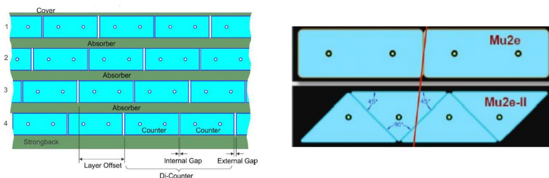
Рис.7. Слева – разрез модуля CRV эксперимента Mu2e. Справа – сравнение вариантов систем CRV, выполненные из стрипов с прямоугольным и треугольным сечением.
