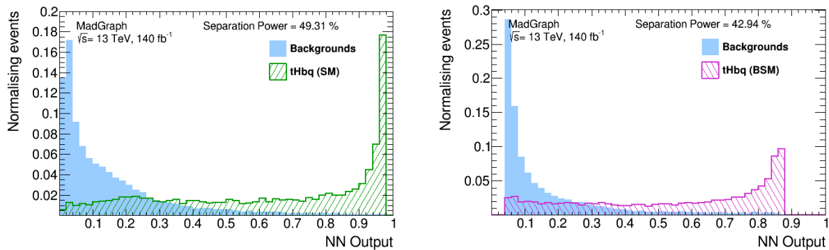
Рис.9. Нормированное распределение отклика сети для тренировочных и тестовых выборок для сигнала СМ(слева) и для сигнала за пределами СМ(справа).
