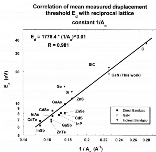
Рис.4. Измеренные значения энергии смещения для различных полупроводников в зависимости от параметра обратной решетки. Большие значения энергии смещения, соответствуют более высокой радиационной стойкости материала [9].
