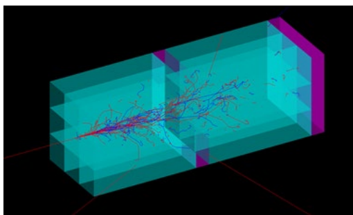
Рис.2. Образец электромагнитного калориметра с моделированными ливнями. Прототип состоит из двух секций, каждая секция собрана из 9 кристаллов PbWO 4 -UF размерами 1x1x4 см 3 .
