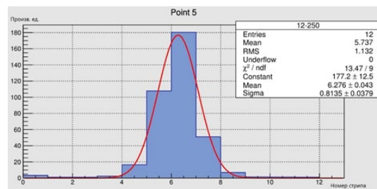
Рис.1. Общий вид строу трубки с внешними стрипами (слева). Распределение сигналов на внешних стрипах при облучении трубки бета источником (справа).
