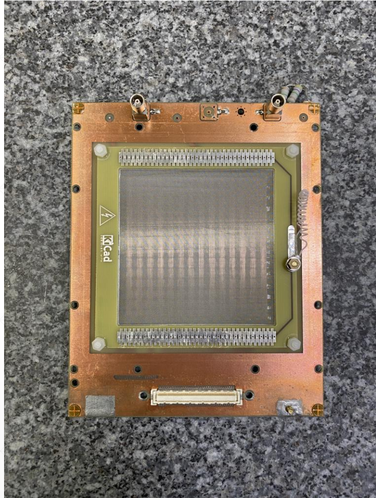
Установка дрейфового зазора
