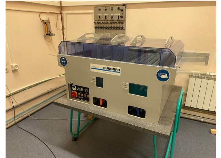
Установка травления
