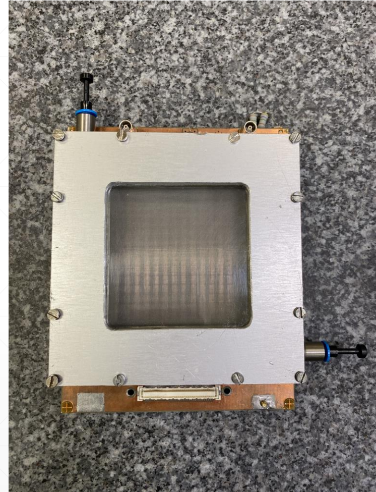
Детектор в сборе
