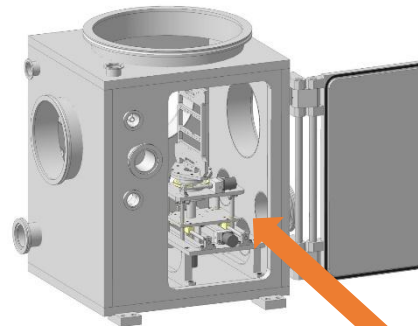
Вакуумная камера на установке СОЧИ @ NICA
