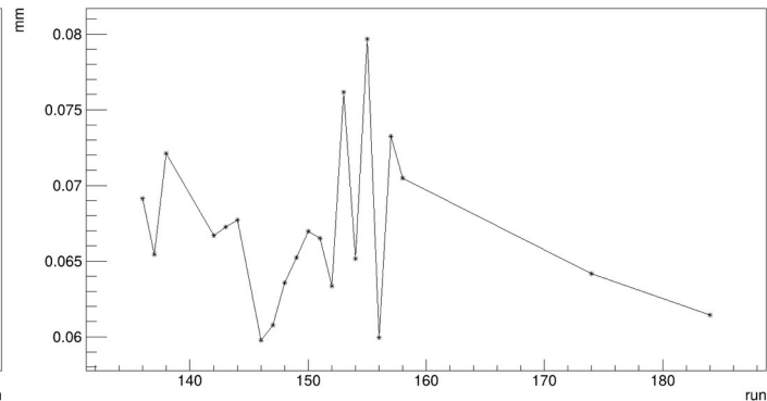
Geometry. Mimosa 1. Shift y
