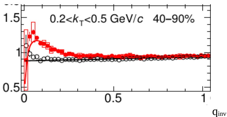
Рис.4. Корреляционная функция пар K^\pm K^\pm в зависимости от q_{inv} . Красные точки — эксперимент, красная кривая — результат модельного фита. кружки — фоновая функция.
