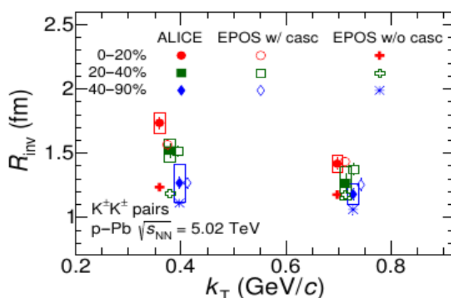
Рис.5. Радиус источника излучения каонов ( R_{inv} ) в зависимости от k_T и центральности событий. Результаты модели EPOS приведены для сравнения.
