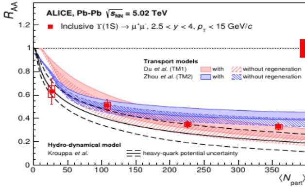
Рис.7. Фактор ядерной модификации ( R_{AA} ) для \Upsilon(1s) , образующихся в Pb-Pb столкновениях при 5.02 TeV с числом нуклонов — участников N_{\text{part}} в сравнении с теоретическими моделями.
