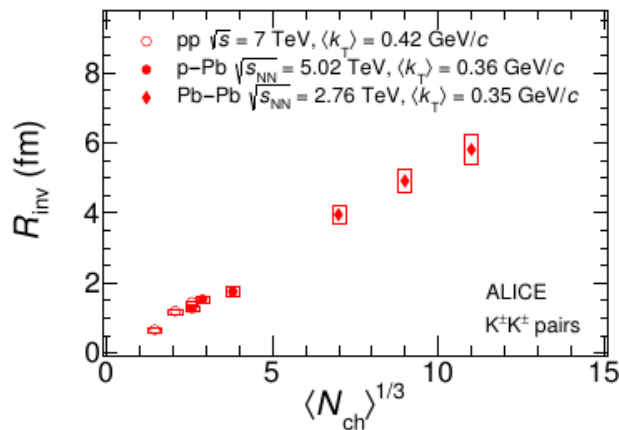
Рис.6. Зависимость R_{inv} для каонов от множественности заряженных частиц ( N_{ch} ) для разных взаимодействующих систем.
