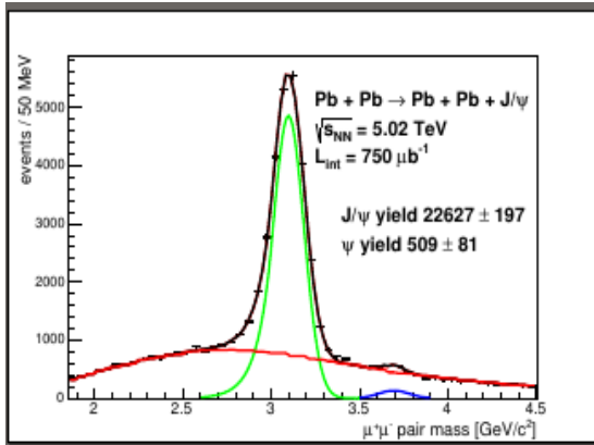
Рис.11. Распределение по инвариантной массе \mu^+\mu^- пар. Кривые линии обозначают разные вклады (смотрите текст).
