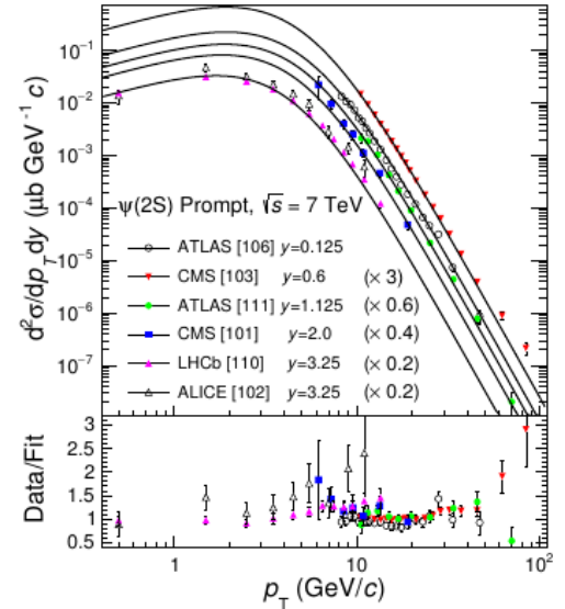
Рис.9. Дифференциальные сечения рождения \psi(2s) в pp при 7 TeV в различных экспериментах. Кривые - результаты фитирования в модели.
