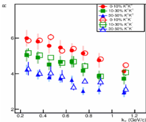
Рис.3. Зависимости радиуса источника излучения пар каонов от поперечного импульса пары для Pb-Pb событий с различными центральностями. Результаты для K^+K^- ( K^+K^+/K^-K^- ) показаны открытыми (сплошными) символами.
